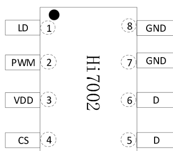
图 5.1 Hi7002 管脚图
